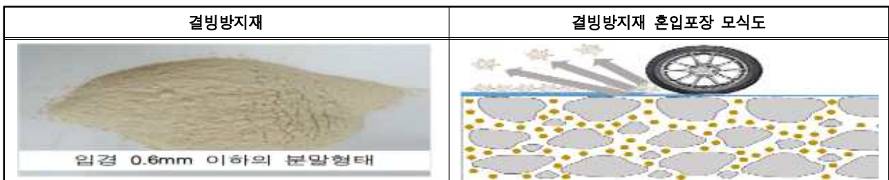
[그림] 결빙방지재 혼입포장 모식도
